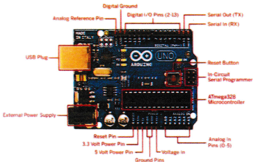
ARDUINO Microcontroller ATmega328
